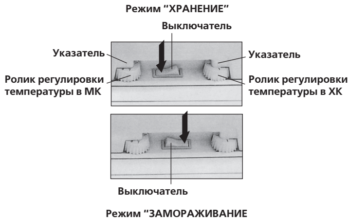
Рисунок 5 — Схема переключения режимов
